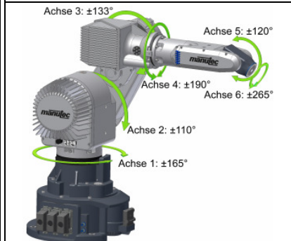
Verfahrbereich Achsen
