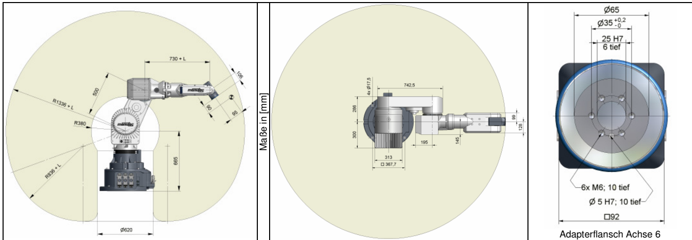
Adapterflansch Achse 6
