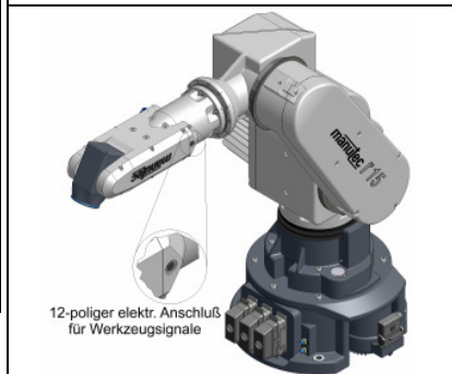
elektrische Anschlüsse 1)
